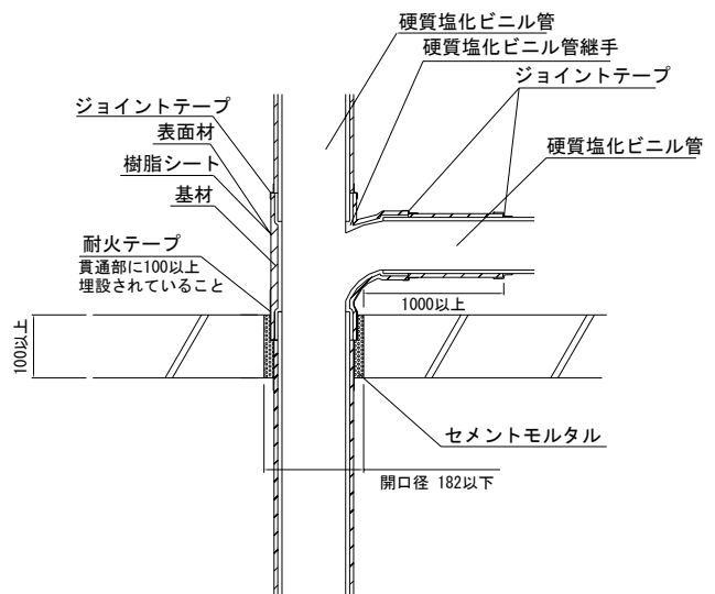
側断面図
