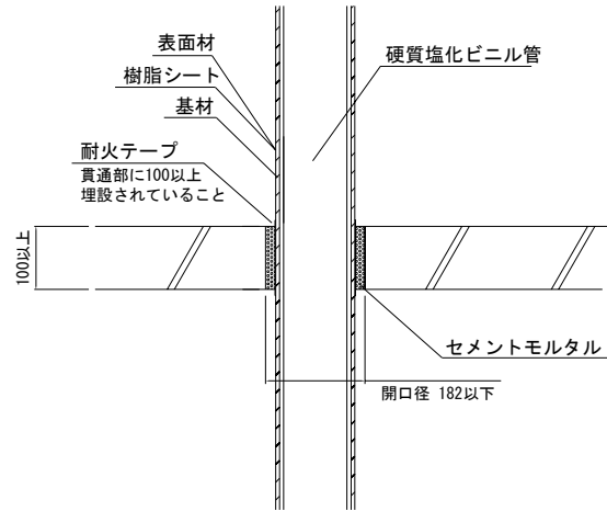
側断面図
